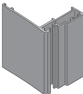
Aile de recouvrement de 70
