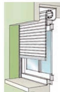
Avec coffre PVC à l'intérieur de la pièce, intégré au bloc fenêtre
